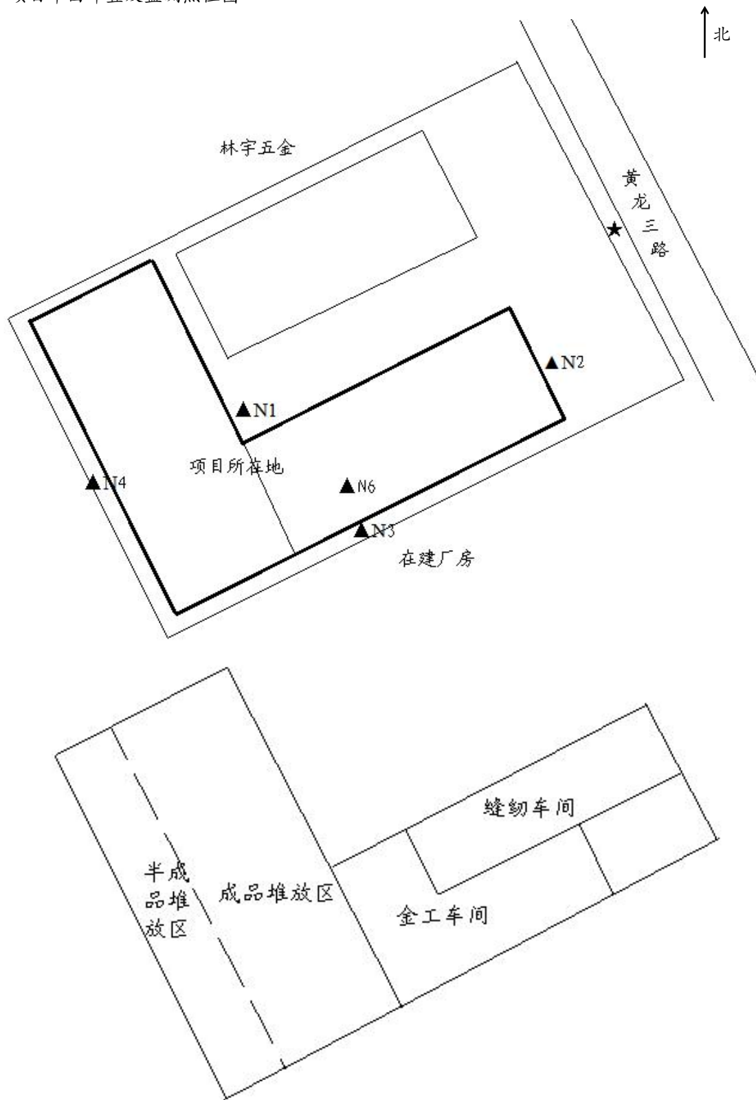
图 3-2 项目平面布置及监测点位图
